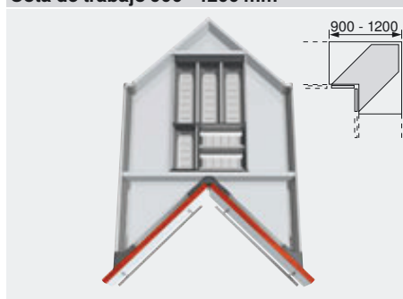
SPACE CORNER Cota de trabajo 900 - 1200 mm
